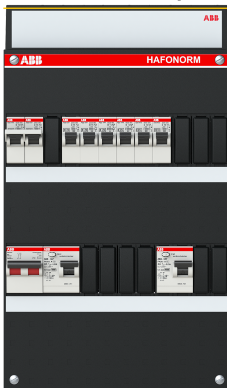
Installatiekast stekerbaar 6 groepen achter 2 aardlekschakelaars 2-pol
