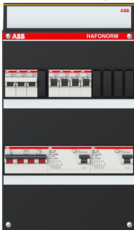
Installatiekast stekerbaar 4 groepen achter 2 aardlekschakelaars 4-pol
