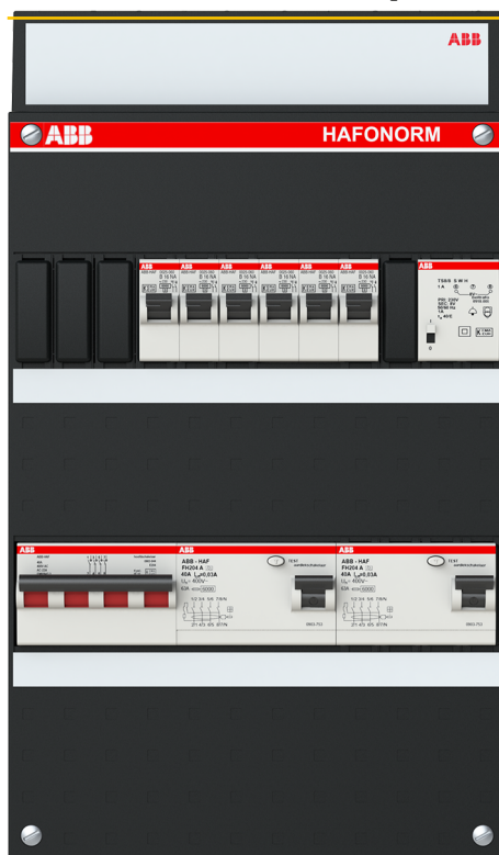
Installatiekast stekerbaar 6 groepen achter 2 aardlekschakelaars 4-pol
