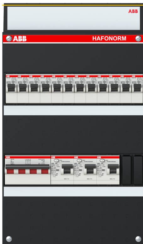
Installatiekast stekerbaar 12 groepen achter 3 aardlekschakelaars 2-po
