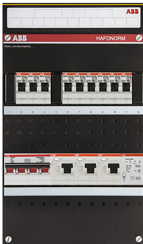
Installatiekast stekerbaar 9 groepen achter 3 aardlekschakelaars 2-pol
